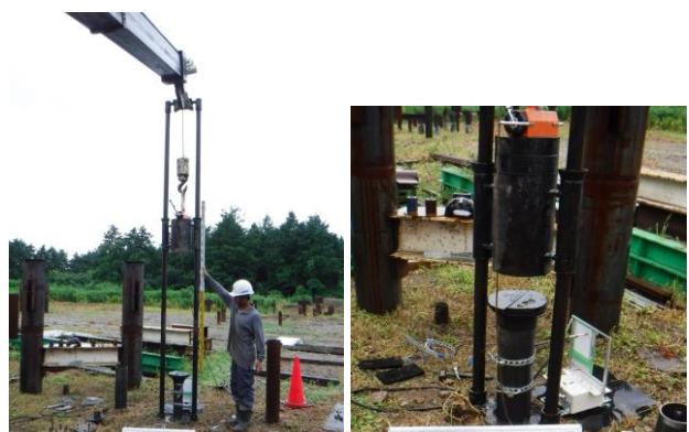
(a) 錘落下高設定状況 (b) 記録状況 写真1 衝撃載荷試験
